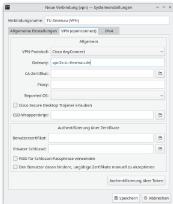
Abbildung 10: Verbindungsnamen und Gateway (vpn2x.tu-ilmenau.de) eintragen
