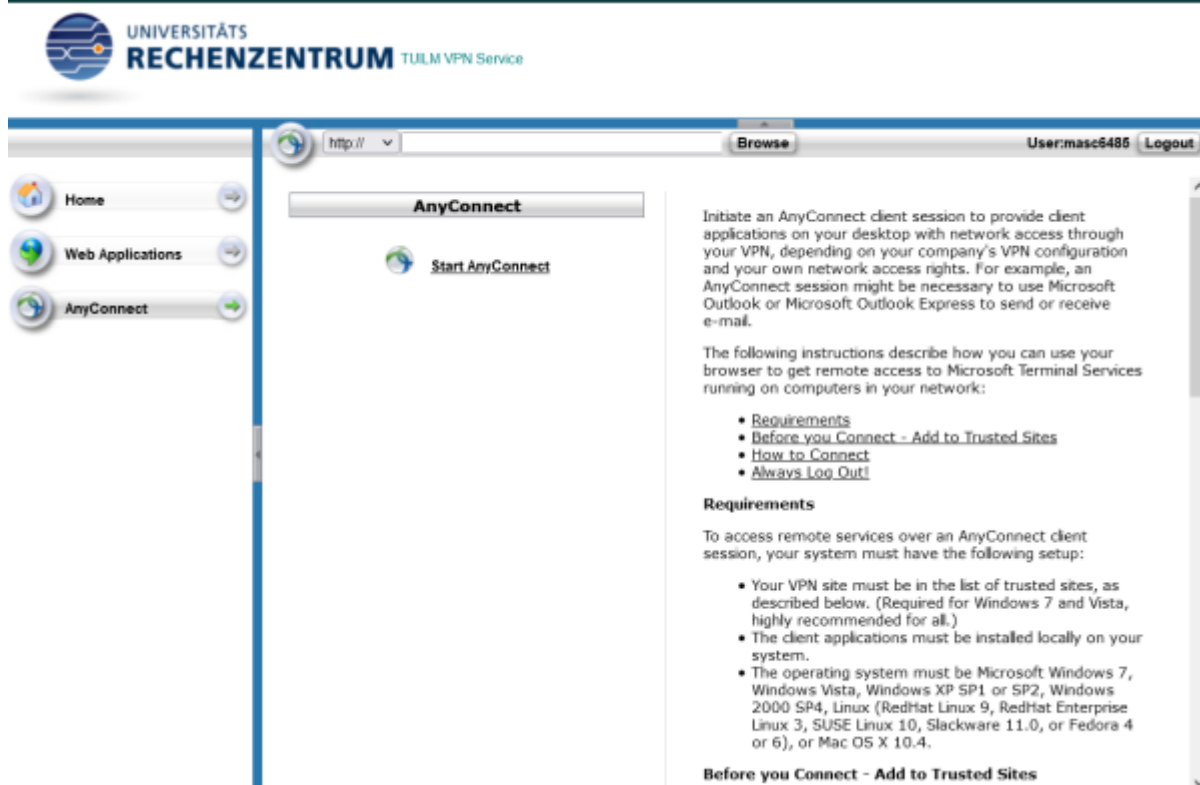
Abbildung 2: Links auf „AnyConnect“ klicken und anschließend auf „Start AnyConnect“
