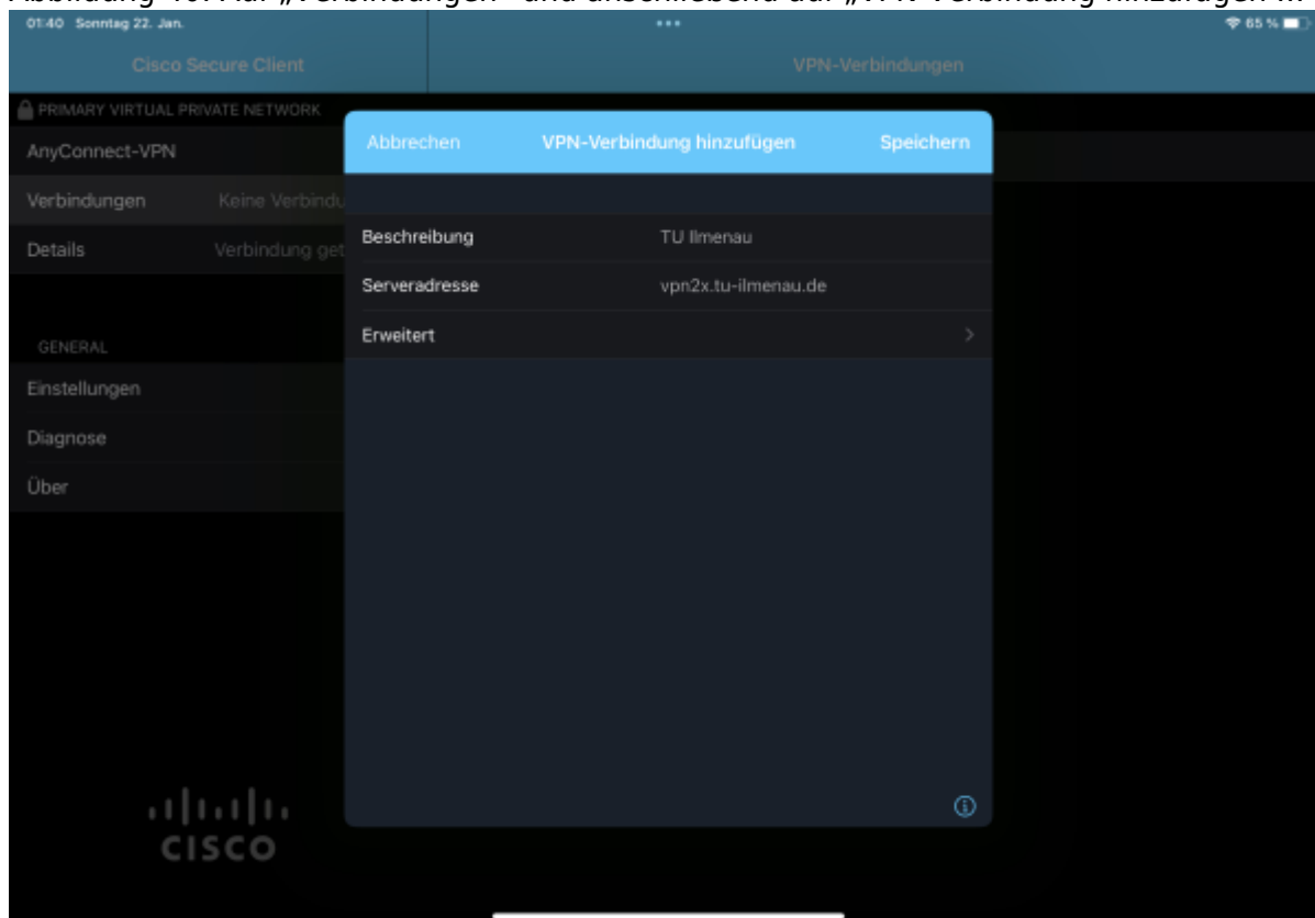
Abbildung 41: Bei „Beschreibung“ einen Titel für die Verbindung und unter „Serveradresse“ die VPN-Server-Adresse vpn2x.tu-ilmenau.de eingeben. Anschließend auf „Speichern“ klicken.
